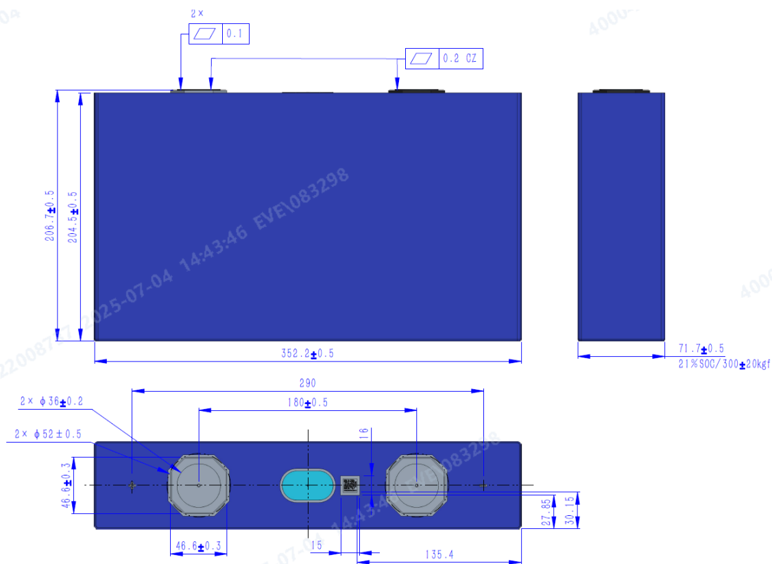
图 8 电池尺寸及外观图 (U 型包膜)
