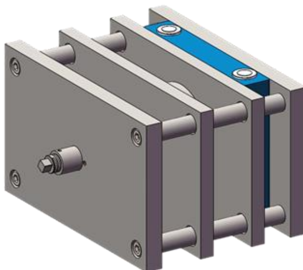
图 6 电池循环夹具图 Fig. 6 Battery Cycling Fixture Schematic
